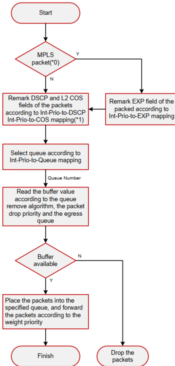
Рисунок 51. Процессы планировки и управления очередями
