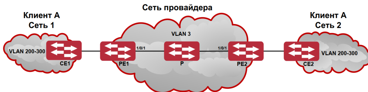
Рисунок 32. Межсетевое взаимодействие на основе Dot1q-туннеля
