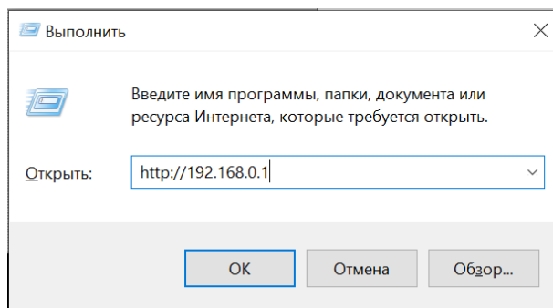
Рисунок 8. Запуск HTTP-протокола
