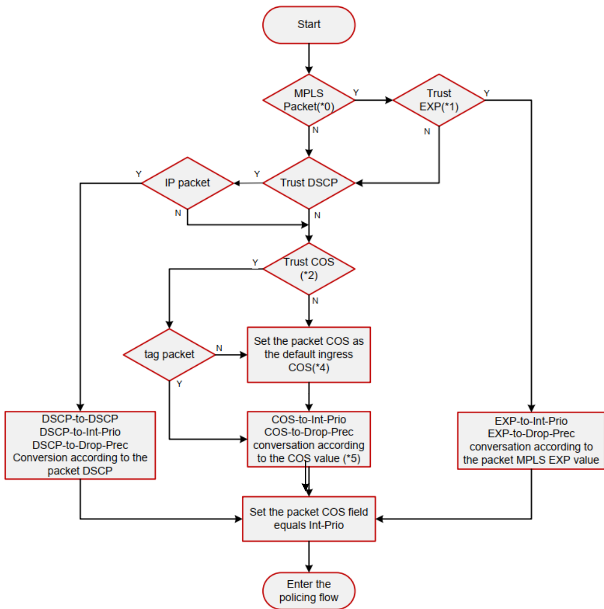
Рисунок 49. Процесс классификации
