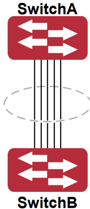
Рисунок 21. Конфигурация Port-Channel
