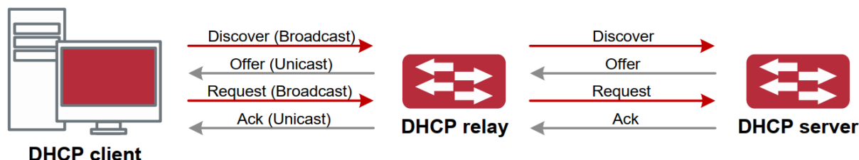
Рисунок 58. DHCP-ретранслятор
